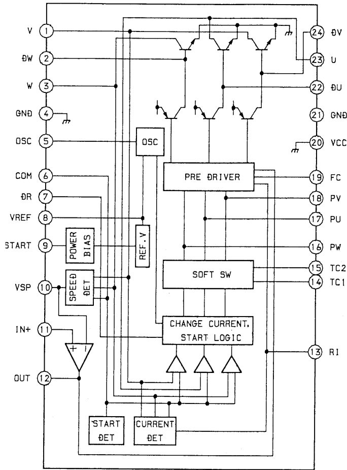
IC601 LB1674V
