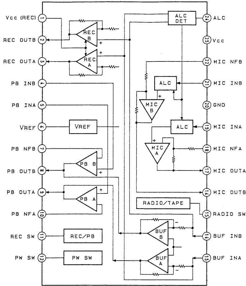
IC101 TA8155FN
