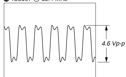
❿ IC3107 ④ 12.4 MHz
