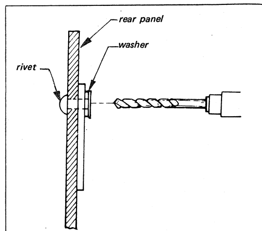
Fig. 2-7. Rivet replacement
