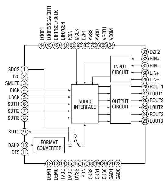
IC605 AK4527
