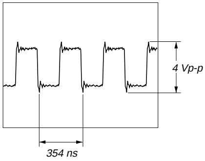
7 IC601 29 (BCKI2), IC604 14 (BCK)
