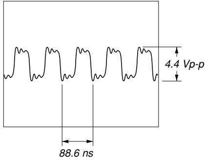
5 IC601 22 (KFSIO), IC604 13 (CKOUT)
