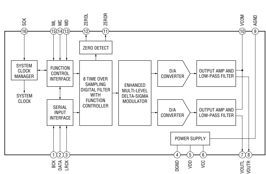
IC606 PCM1748E/2K
