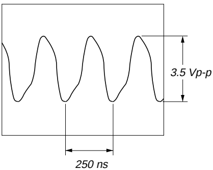
1 IC601 23 (XOUT)
