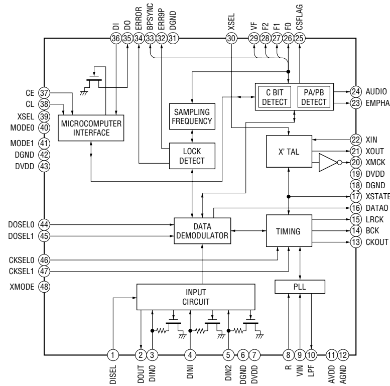
IC604 LC89056W-E
