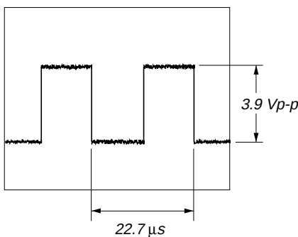
6 IC601 28 (LRCKI2), IC604 15 (LRCK)
