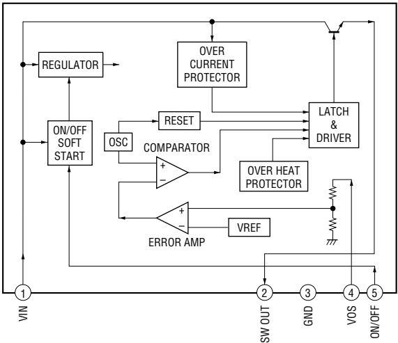
IC1405 SI-8120JF
