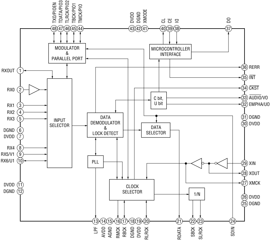
IC2208 LC89057W-VF4A-E
