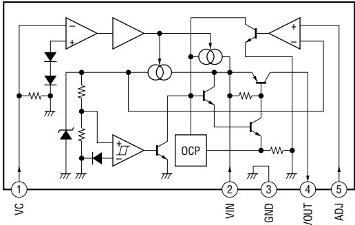
IC2494 SI-3011ZD-TL
