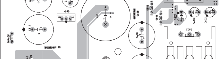
【PS BOARD】(SIDE A)
