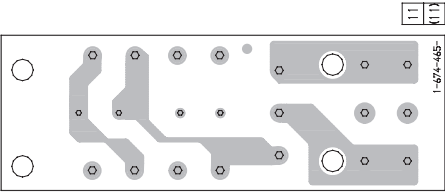
【AC BOARD】(SIDE B)
