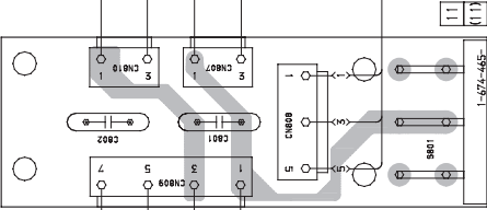
【AC BOARD】(SIDE A)
