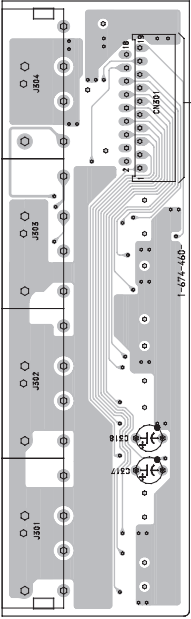
【CN3 BOARD】(SIDE A)
