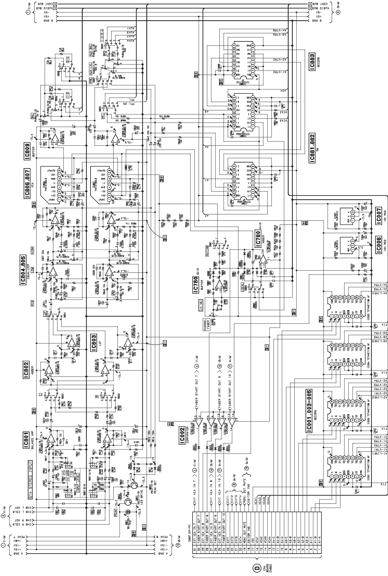
【 MASTER BOARD 】 (2/6)
