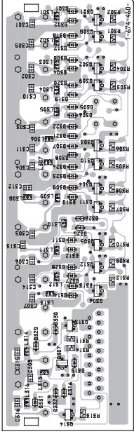
【CN3 BOARD】(SIDE B)
