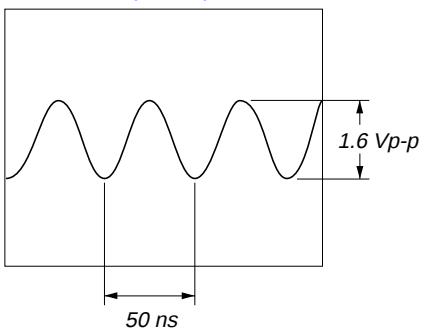
20 IC901 41 (EXTAL)
