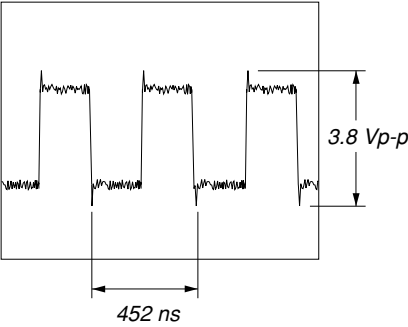
② IC801 ⑤② (OSCI)
