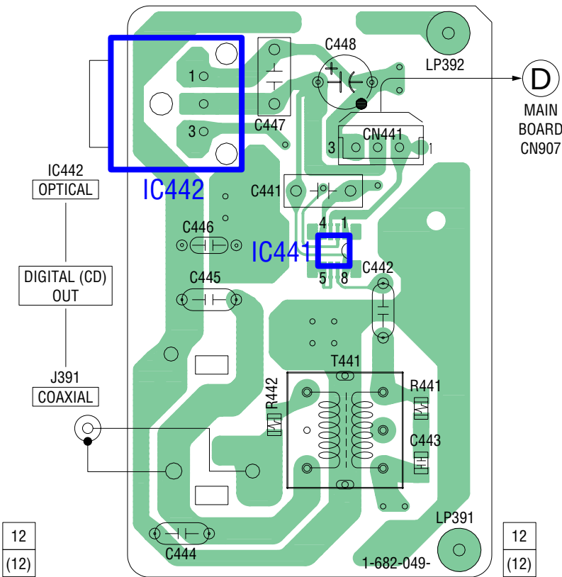
【D.OUT BOARD】(CONDUCTOR SIDE)
