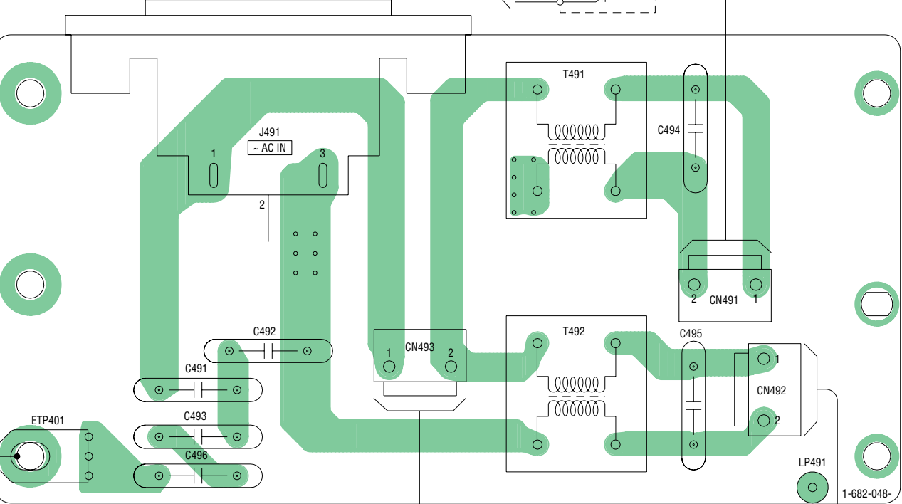
【AC BOARD】(CONDUCTOR SIDE)
