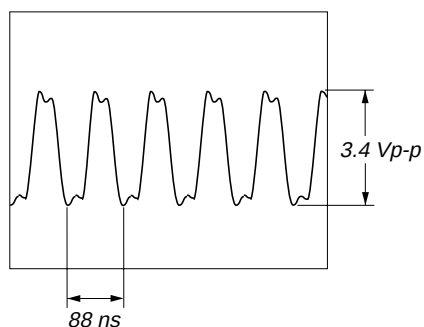
⑩ IC901 ④① (EXTAL)
