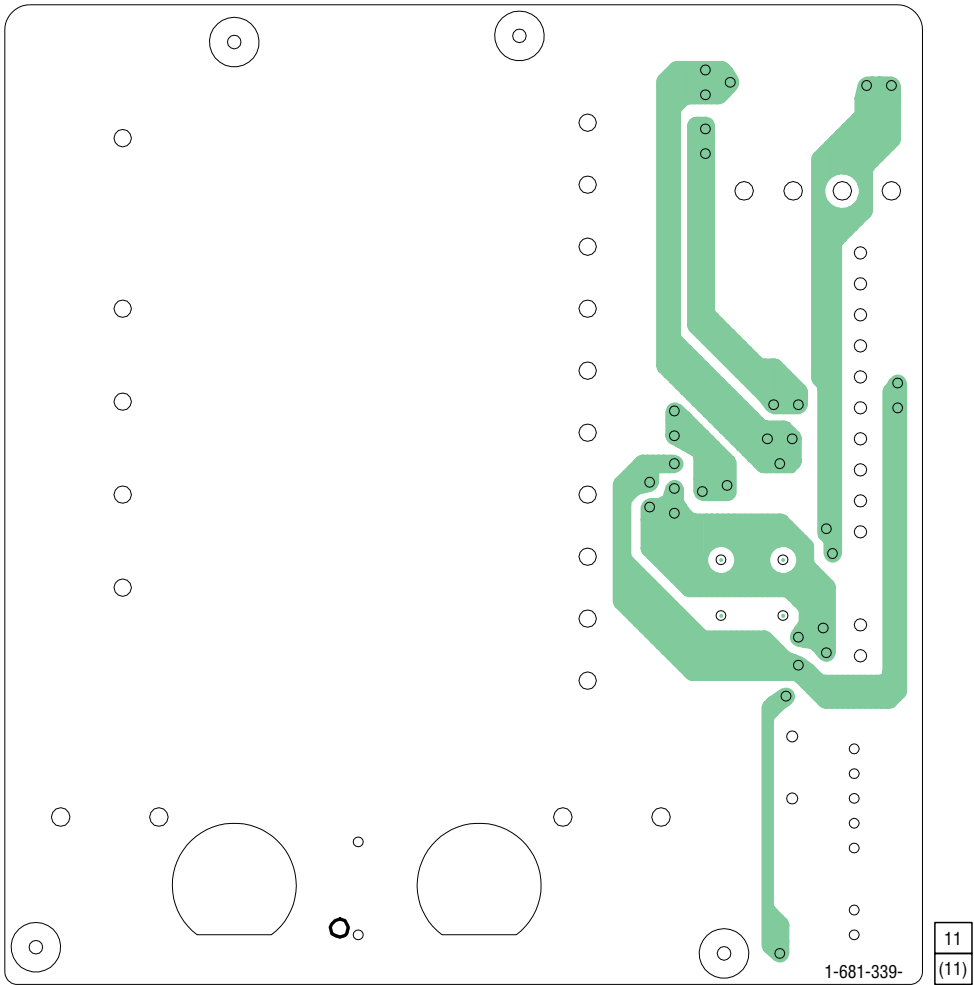
【PT BOARD】 (COMPONENT SIDE)
