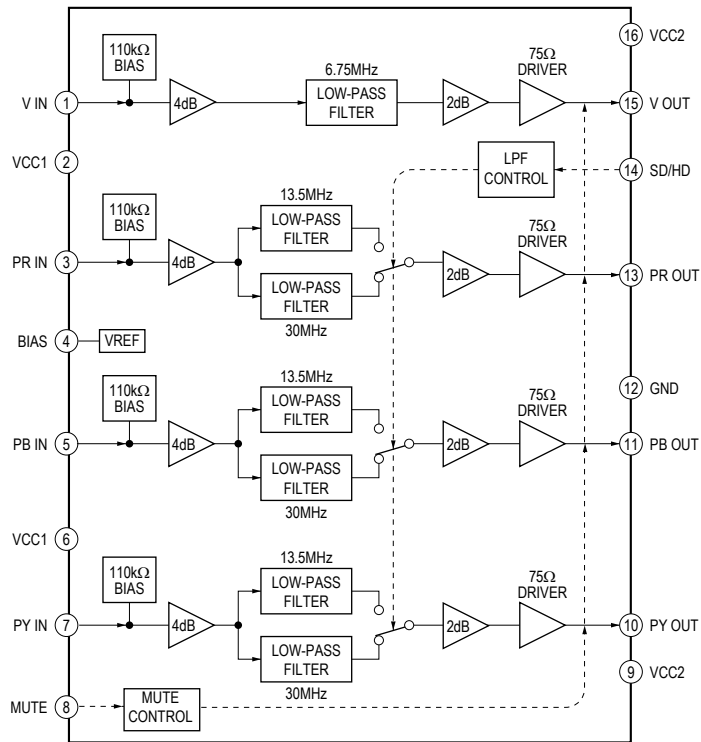
IC1003 MM1797CVBE
