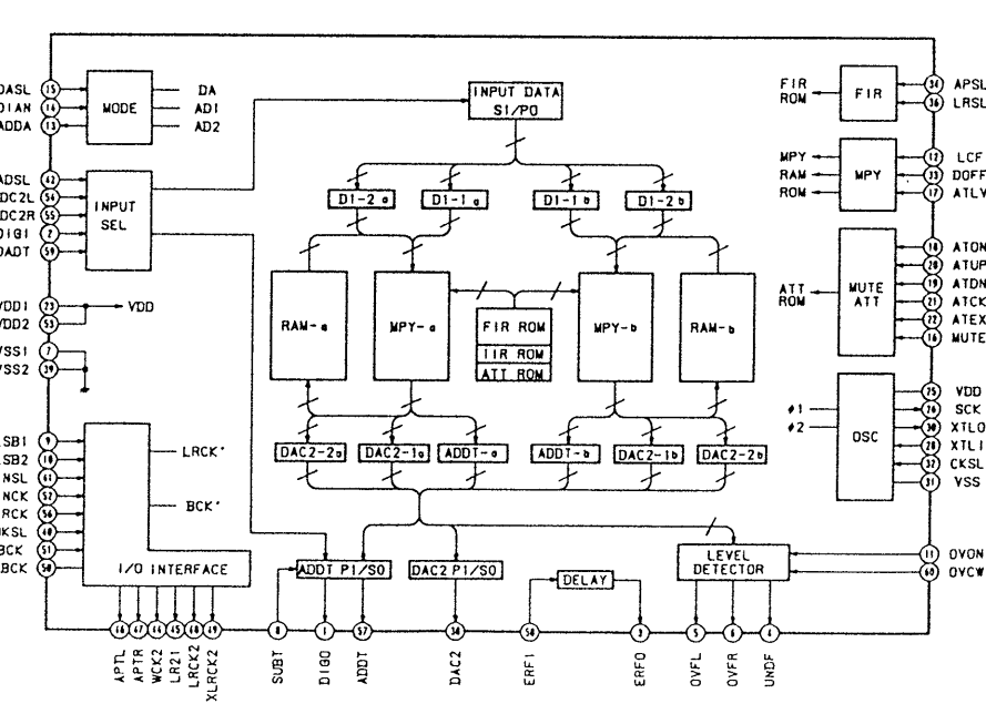
IC306 CXD1136Q
