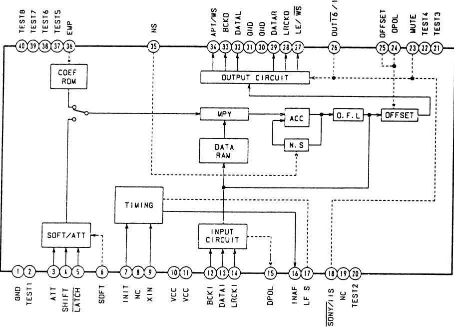
IC802 BX-1387
