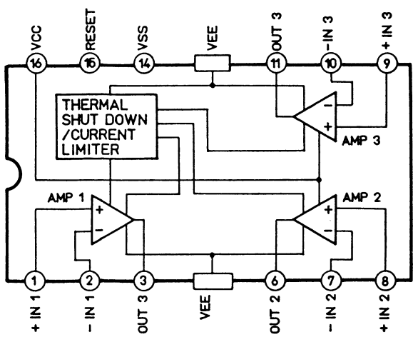
IC102, 103, 105 LA6523
