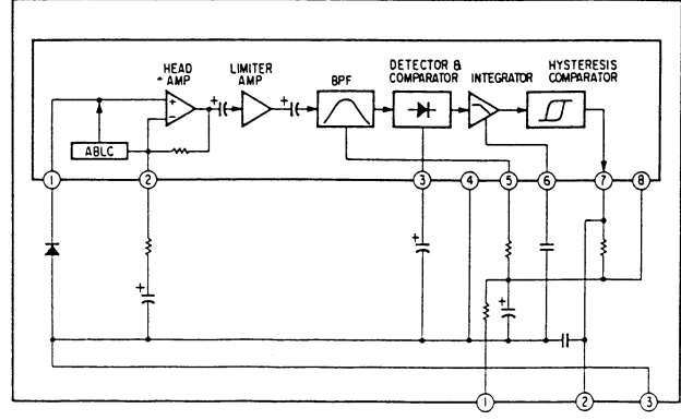
IC802 BX-1387
