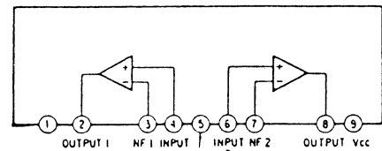
IC304 CXD2557M
