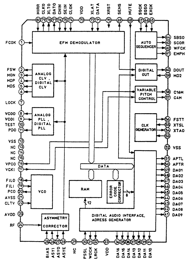
IC201 CXD2500Q
