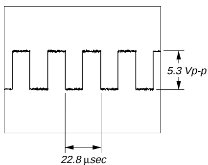
❹ IC105 ④⑤ (LRCK)
