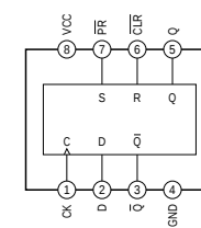
IC303 TC7W74FU
