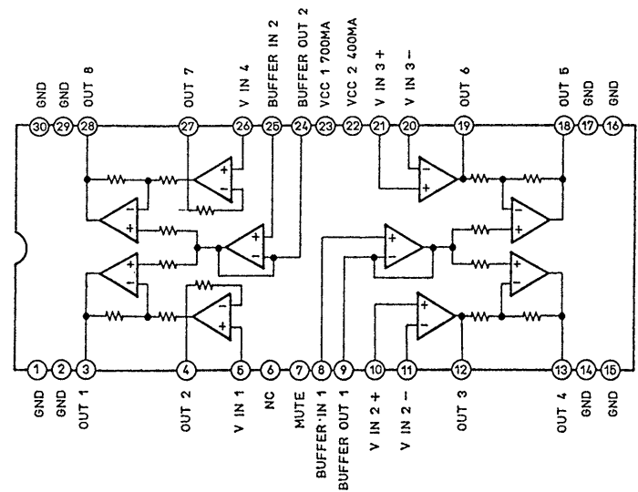
LA6532
