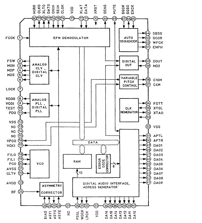
CXD2500
