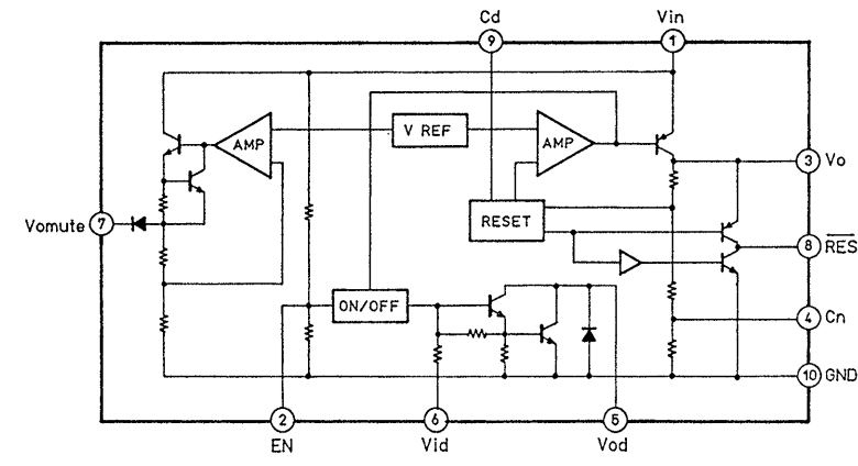
LA5601
