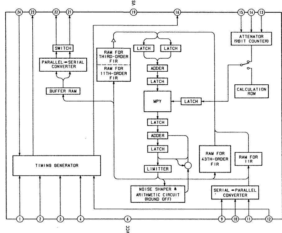
CXD2551M
