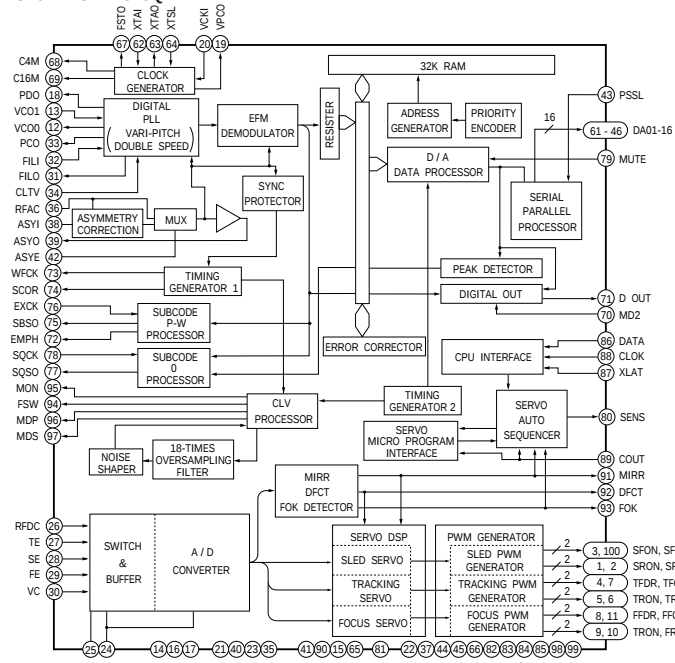
IC101 CXD25450
