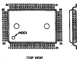
LA5602
