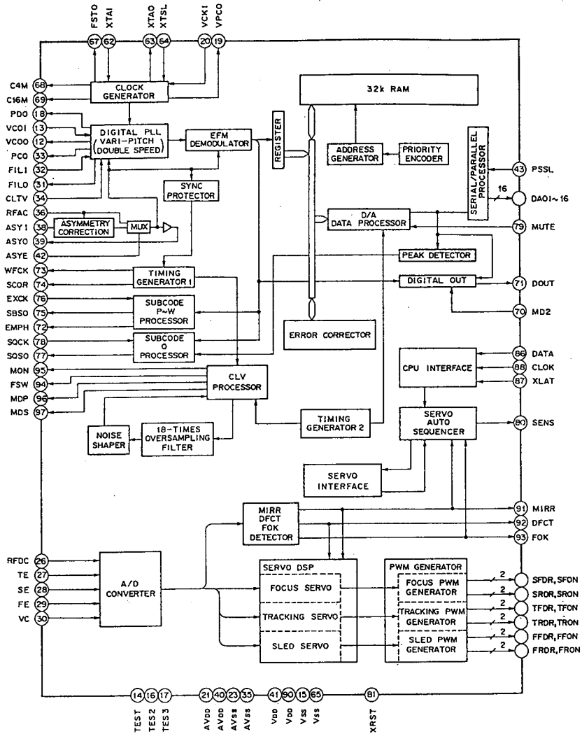
IC101 CXD2515Q/2599Q
