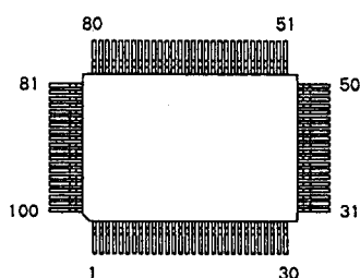
CXD25605M-T6
