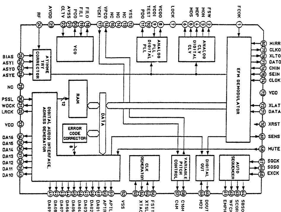
IC301 CXD2500Q
