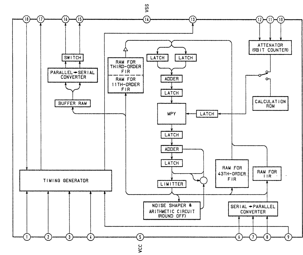
IC304 CXD2551P
