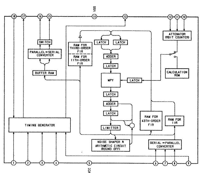
IC302 CXD2551P
