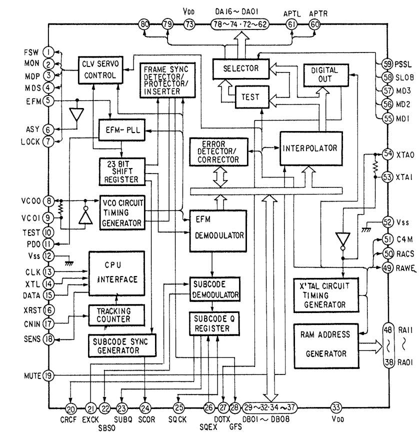
IC301 CXD1125Q
