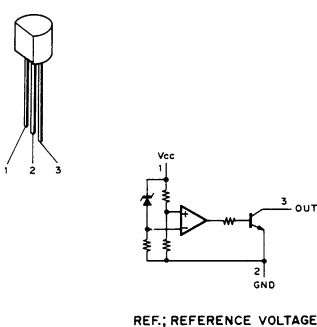
PST520C (MITSUMI) 4.5V SYSTEM RESETING DEVICE
