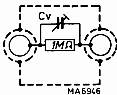
Fig. 3.22. 2:1 Dummy probe
