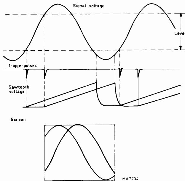
Abb. 2.4. Abtasten der Wellenform mittels des LEVEL Potentiometers
