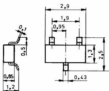
SOT-23
