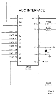
Fig. 2.13. ADC interface
