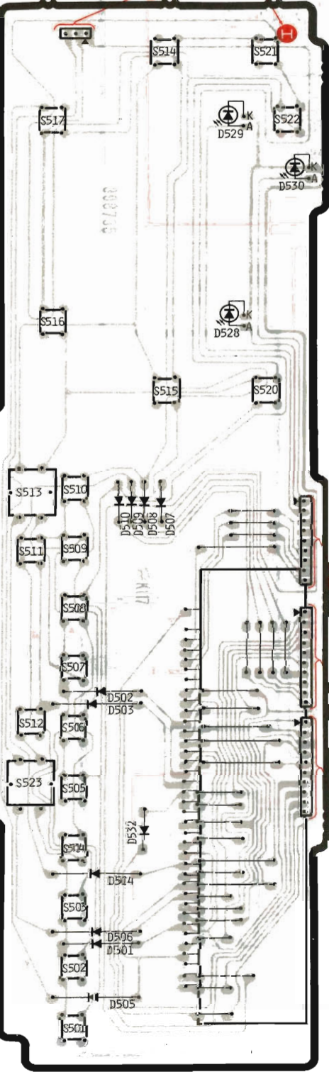
CONTROL P.W.B.
