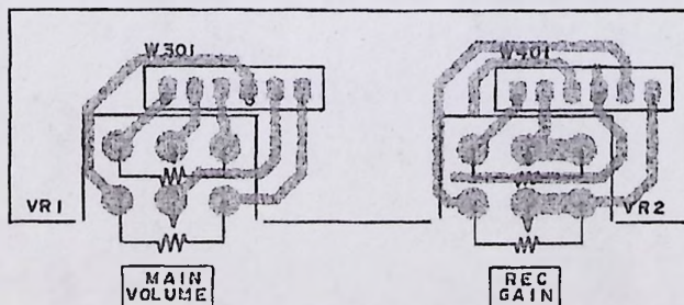
VOLUME PCB L6036A502E
