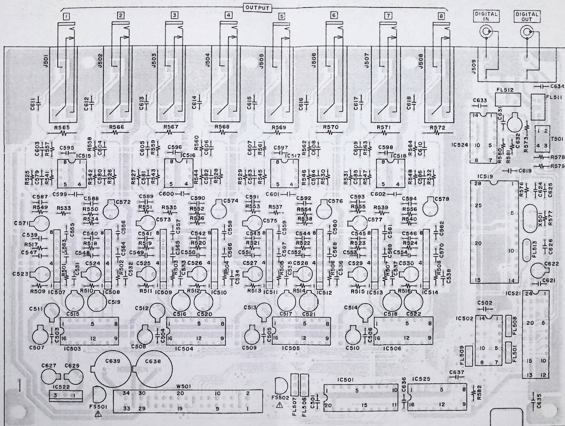
8 PARA/DIO PCB L6036A501A
