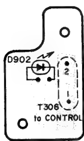
ディテクター(B)基板 DETECTOR(B) PCB CMROID1620
