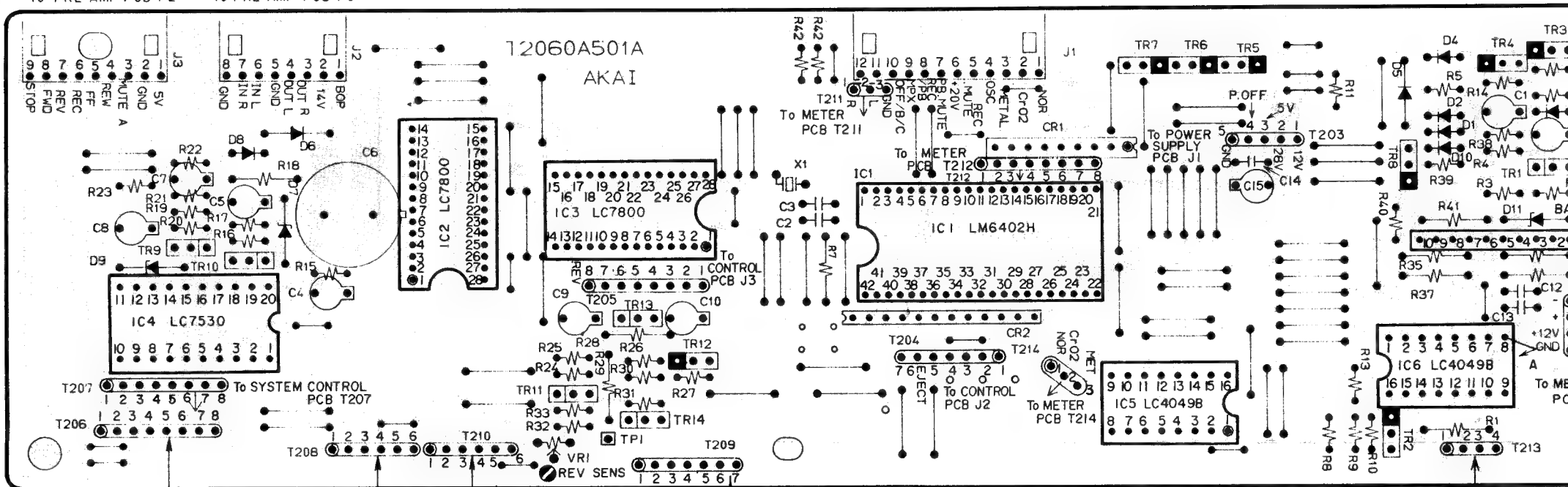
SYSTEM CONTROL PCB T2060A501A システムコントロール基板
