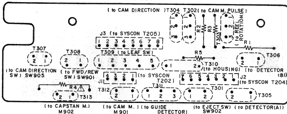
コントロール基板 CONTROL PCB CMROIC189A
