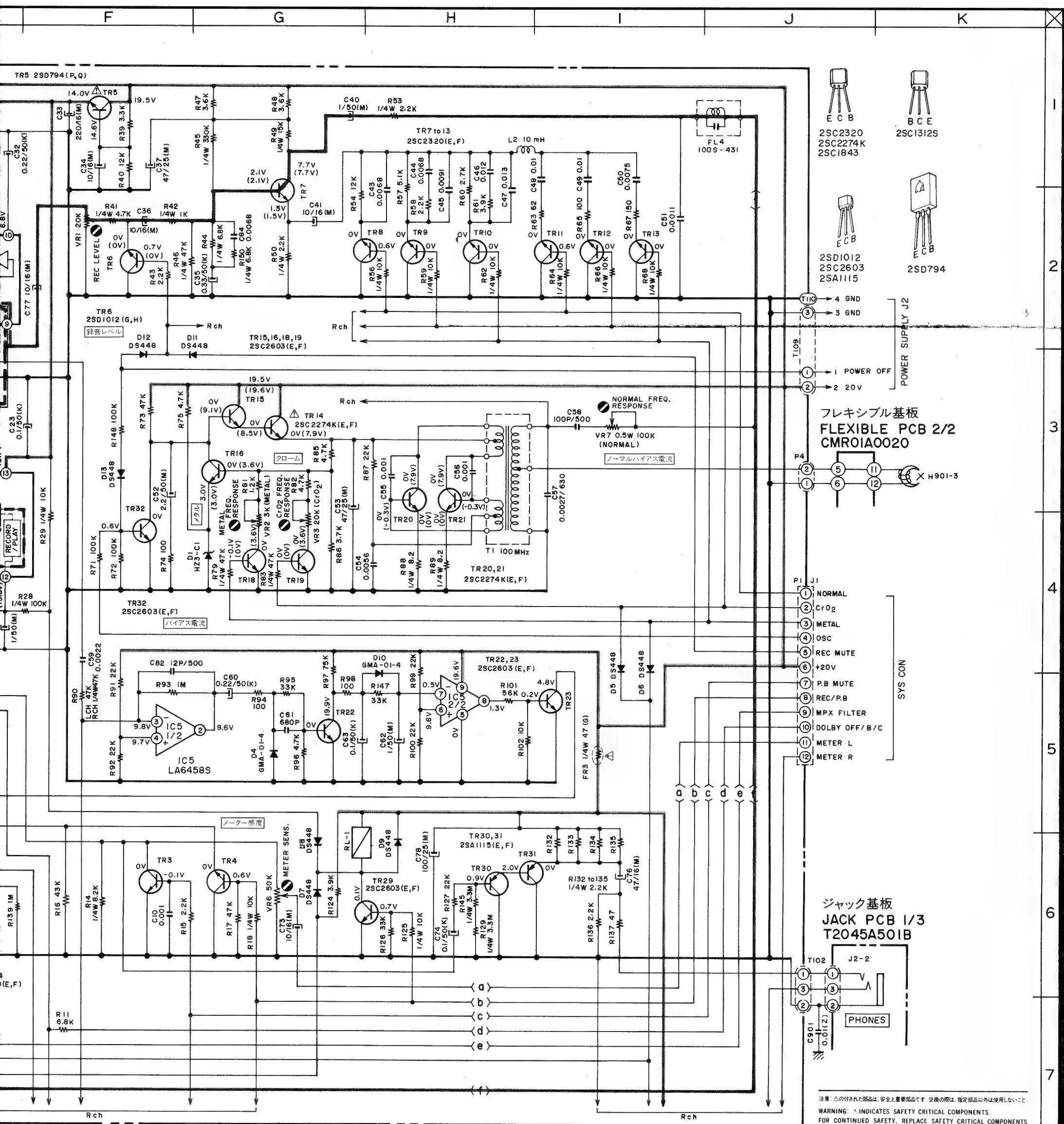
PRE-AMP PCB T2045A501A プリ アンプ基板
