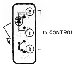
ガイドディテクター基板 GUIDE DETECTOR PCB CMROID0220
