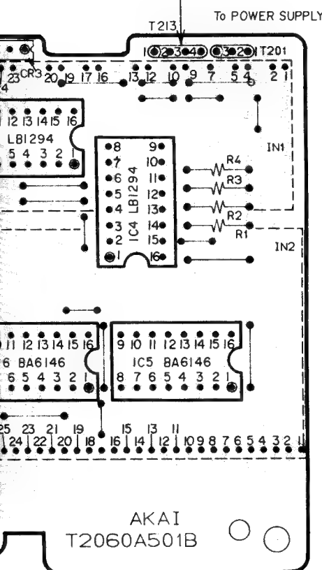
METER PCB T2060A501B メーター基板
