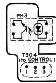
カムディレクション 基板 COM DIRECTION PCB CMROIC189B
