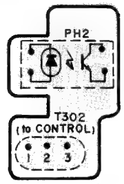
カムモーター パルス基板 CAM MOTOR PULSE PCB CMROIC189C
