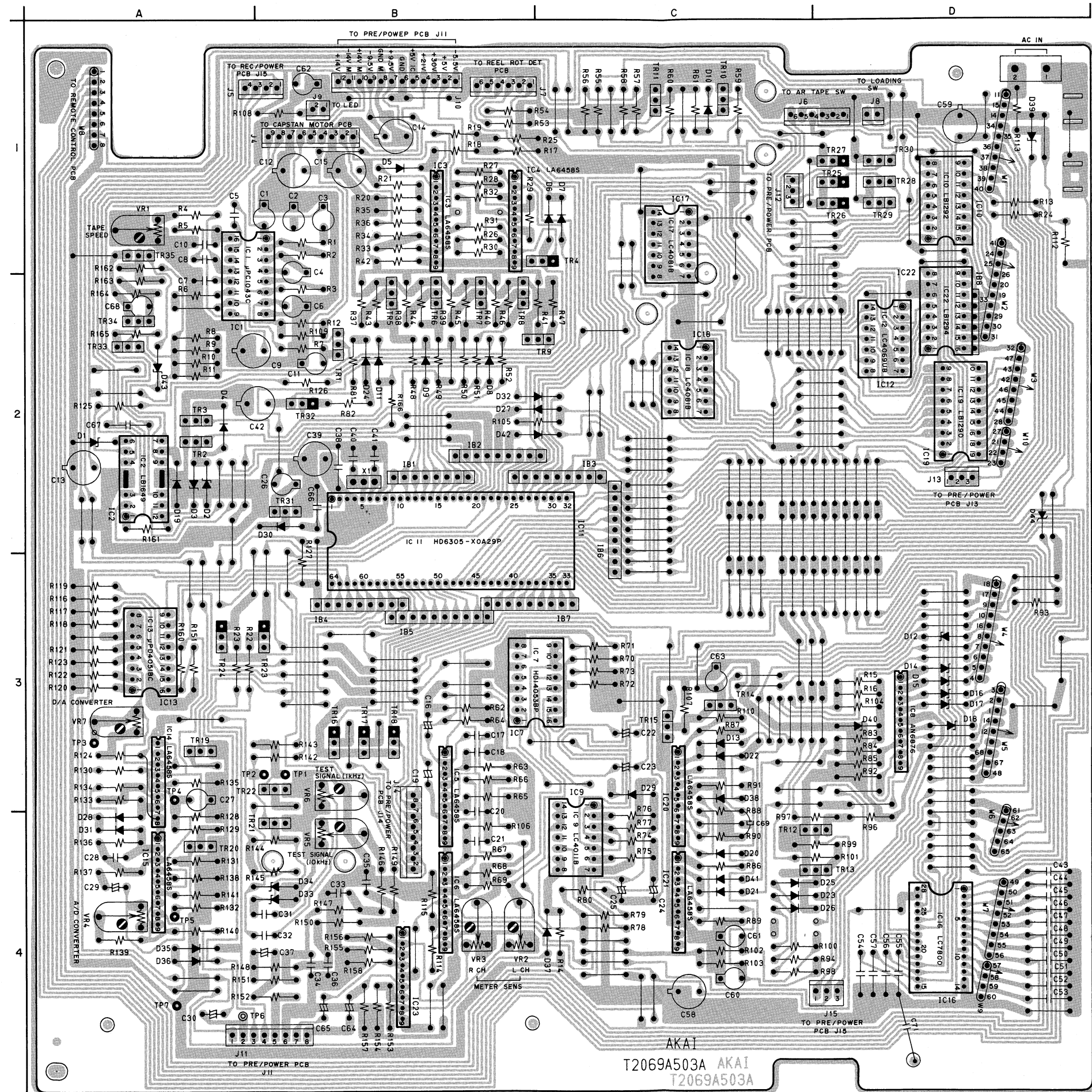
SYSCON/TUNING PCB T2069A503A シスコン・チューニング基板
