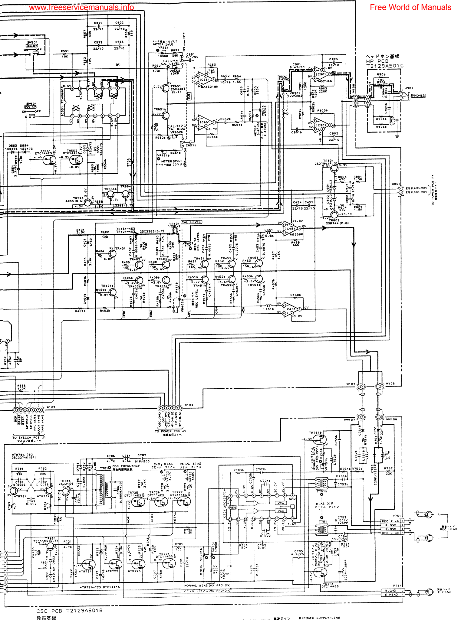
GX-75MKII/95MKII PRE AMP & OSC SCHEMATIC DIAGRAM NO.3-3 T212806M
