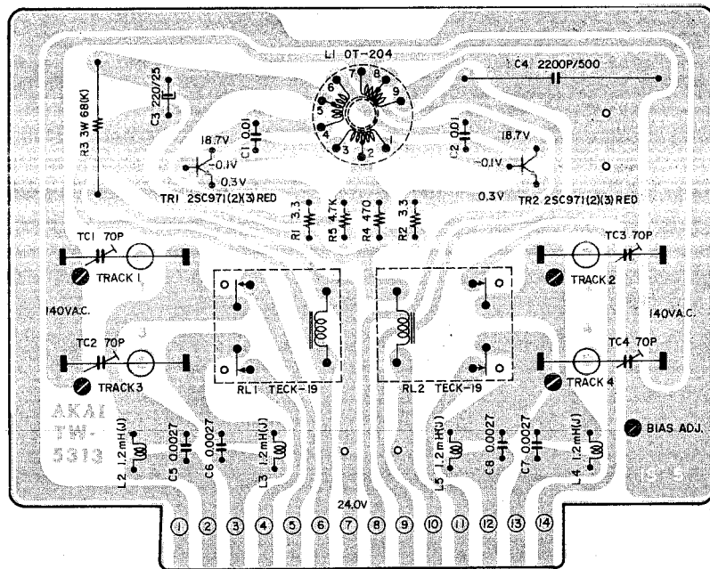
Fig. 12 OSC. P.C. BOARD TW-5313 (REVERSE)
