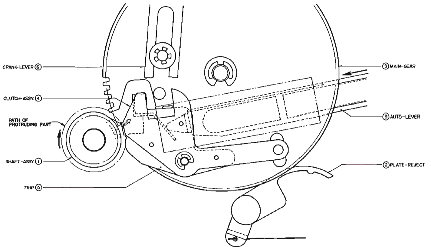
Fig. 10 NON RETURN CONDITION
