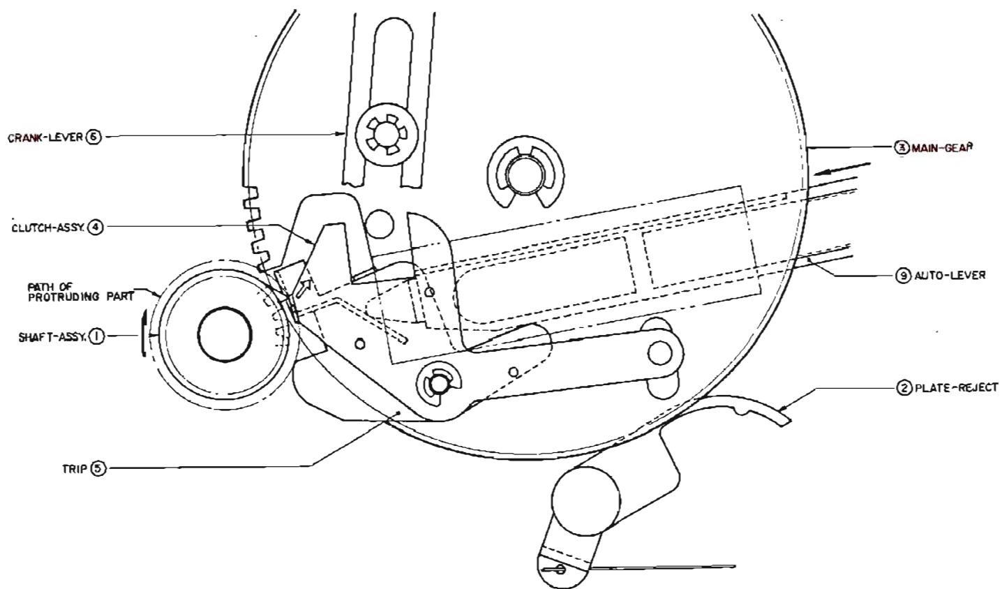
Fig. 12 NON RETURN CONDITION
