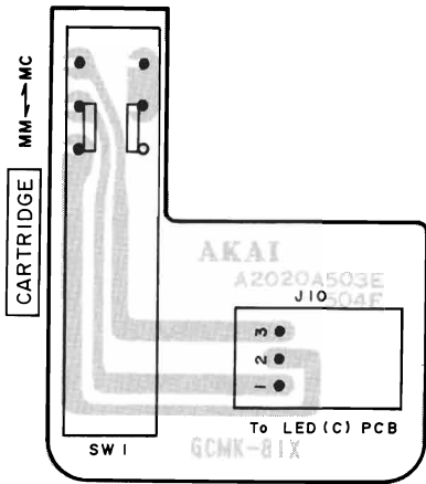
SWITCH PCB A2020A504E
