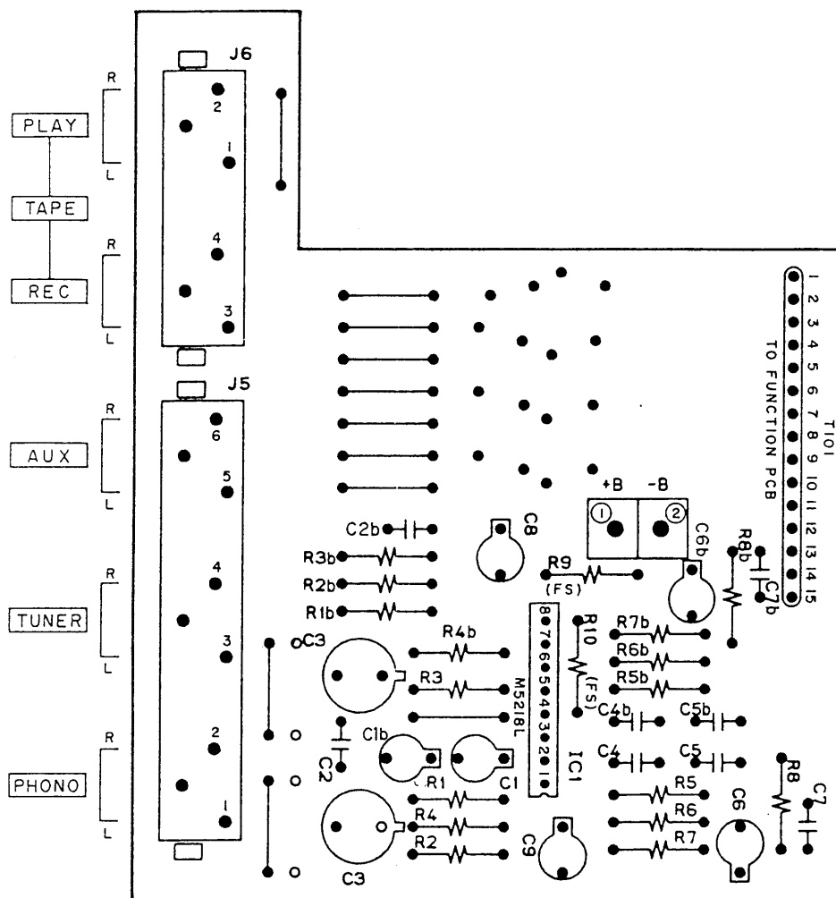
EQUALIZER PCB A2027A501B U,A,C 502B E,B,S
