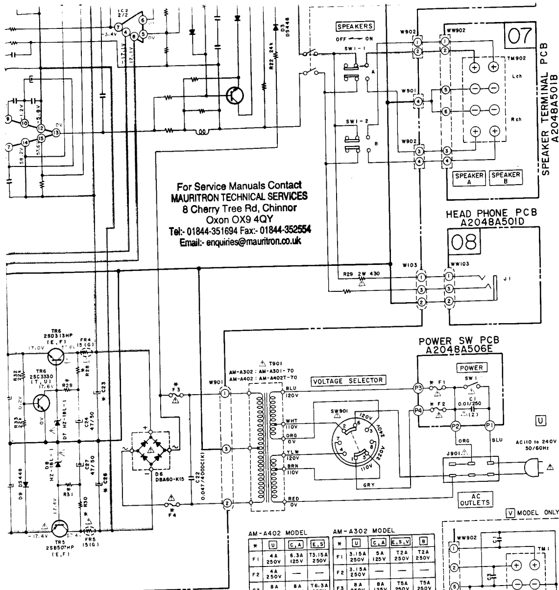
PCB A2048A501A
