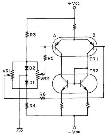
Fig. 5 D.C Balance
