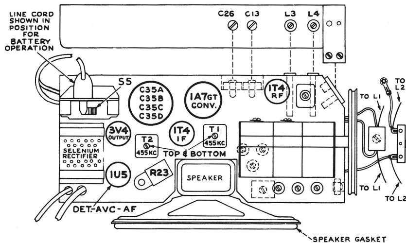
FIG. 1—CHASSIS LAYOUT
