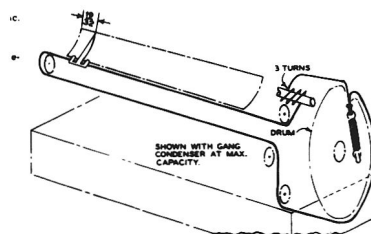
FIG. 7—DIAL CORD STRINGING
