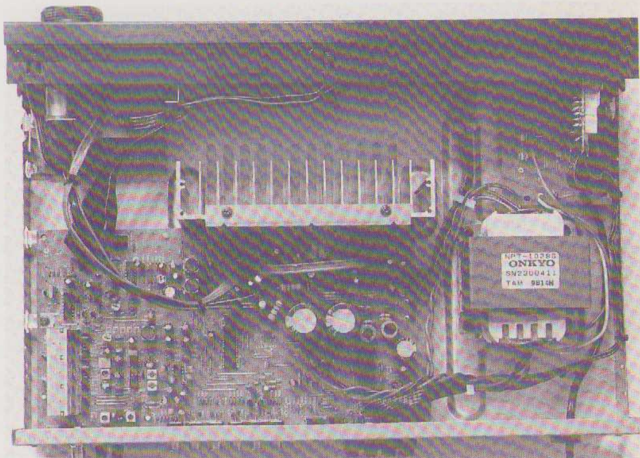
Het binnenwerk van de Onkyo receiver.
