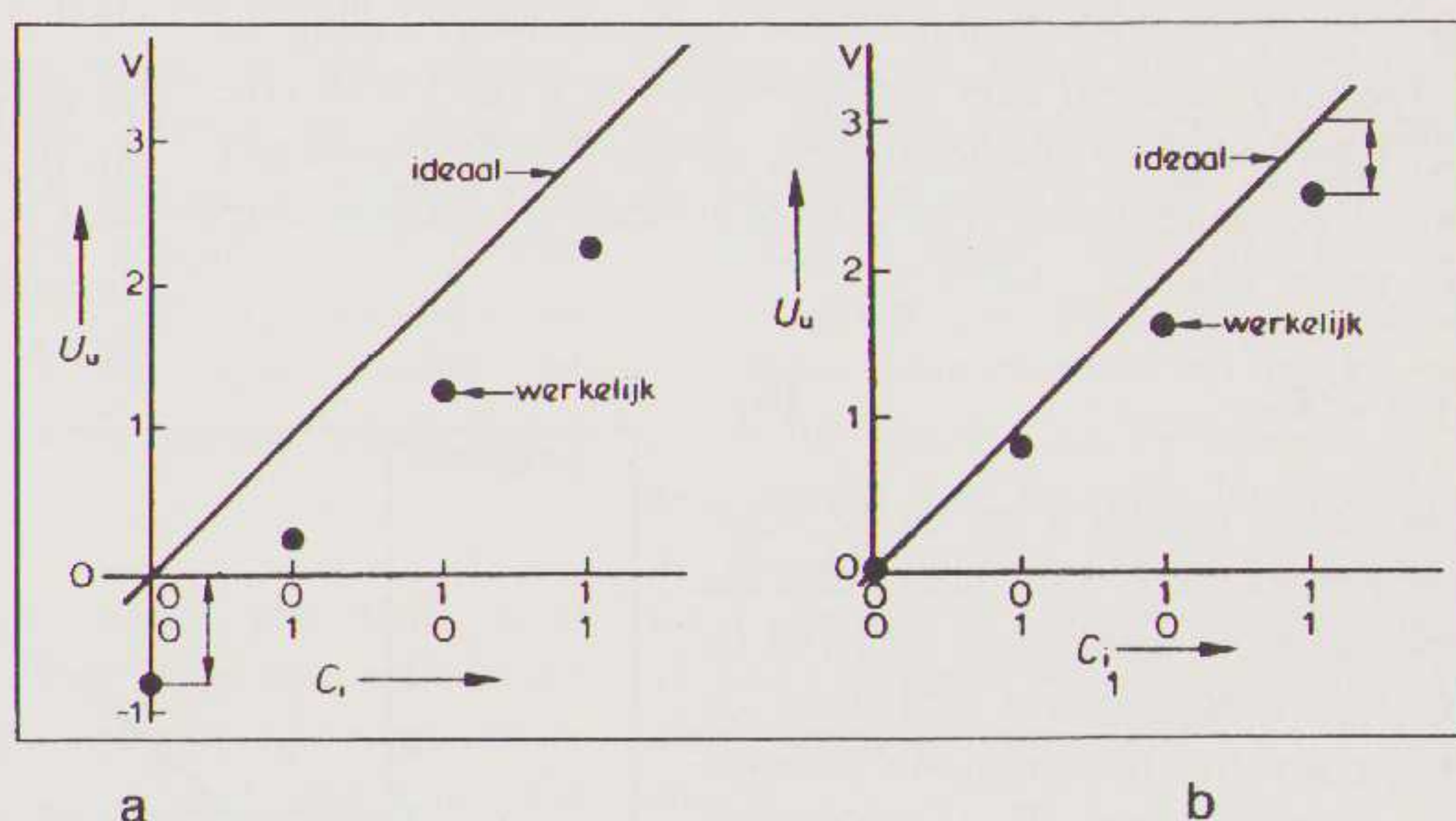
Fig. 9. Overdrachtskarakteristiek van een D/A-converter met een nulfout (a) en een schaalfout (b).
